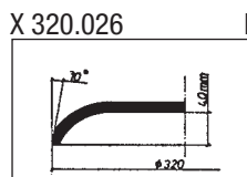
X 320.026 Kienzle 08 42,46
