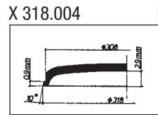
X 318.004 Zentra
