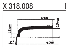
X 318.008 Junghans 93/1954
