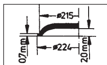
Diehl 42.197-0563
