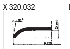
X 320.032 Kienzle 840 4700
