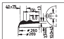
Westend Modell 64
