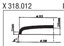
X 318.012 Aristo
