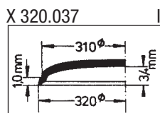
X 320.037 Junghans
